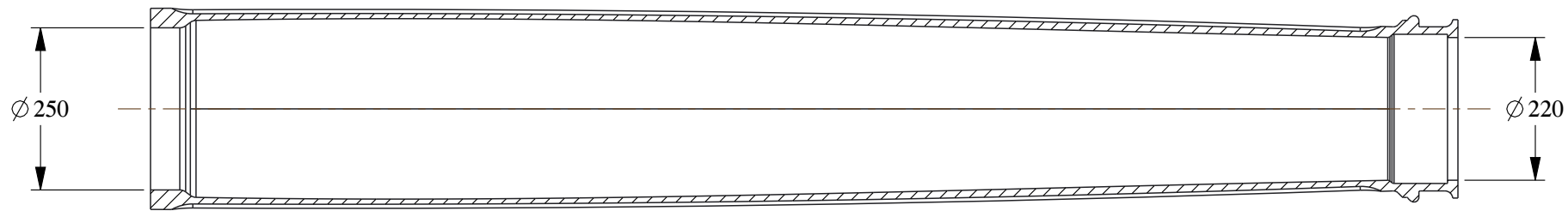
SECTION A-A
